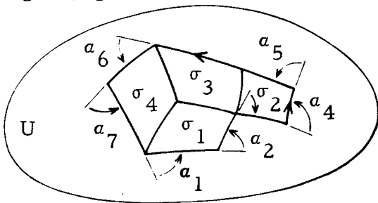
Fig. 8.2 Fundamental Set
