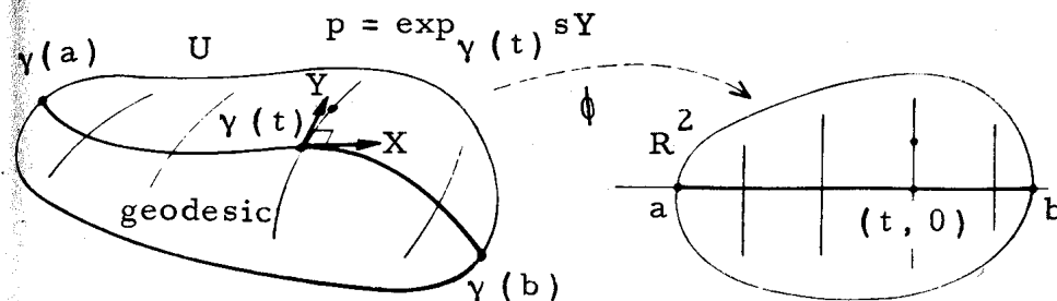
Fig. 9.1 Fermi Coordinates
