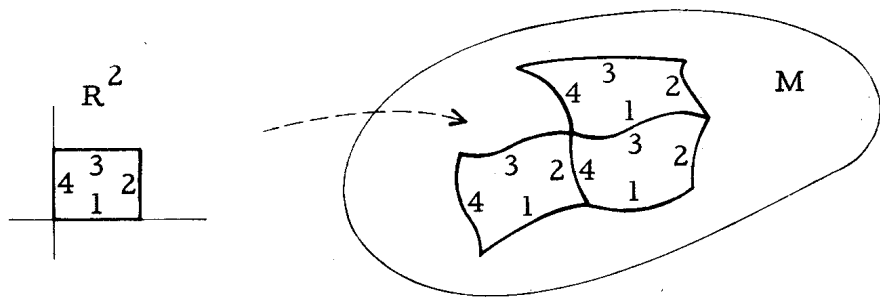
Fig. 7.1. A Fundamental 2-Chain
