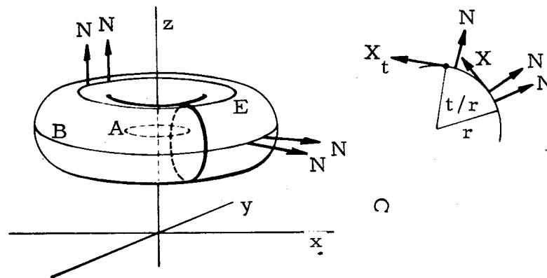
Fig. 2.4 The Torus
